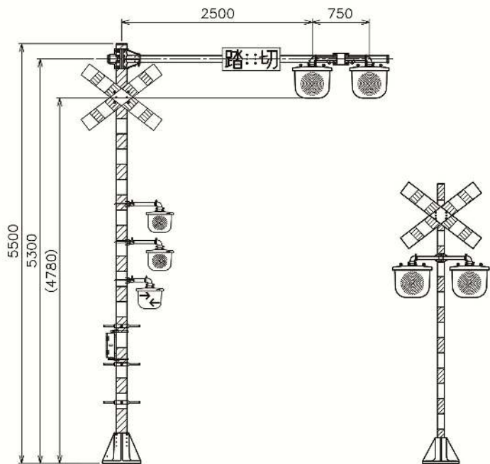
【踏切警報機(OH-AL形)取付例】 【踏切警報機(A形)取付例】
