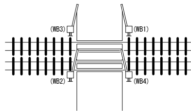
【結線図(複線区間で遮断機が4門の場合)】
