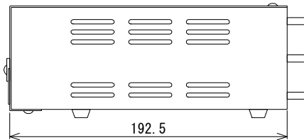
【外観図】
