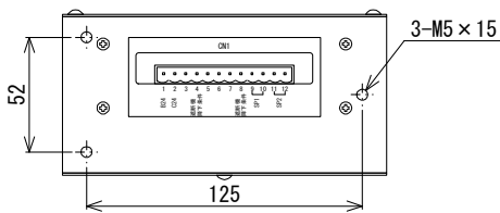
背面図
