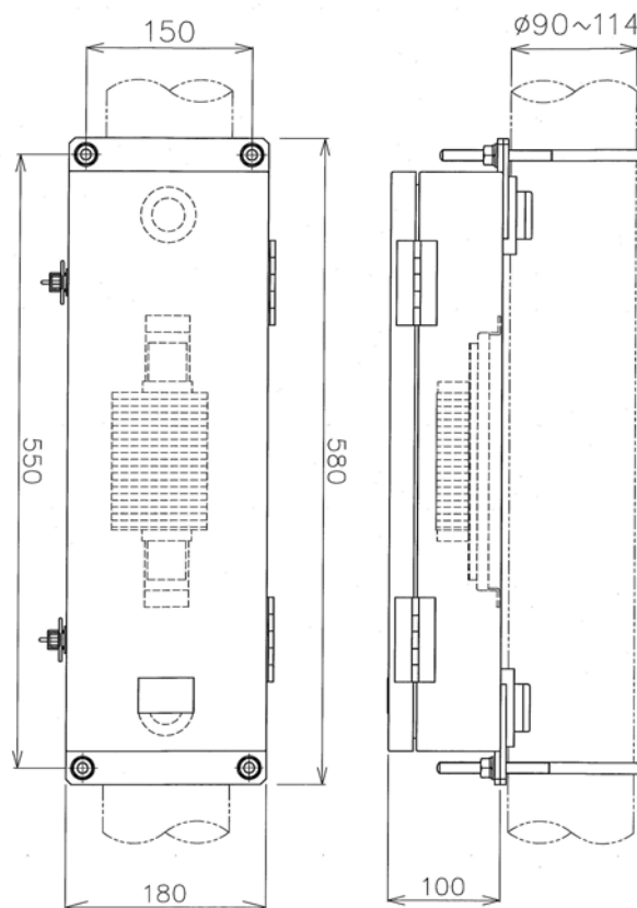
【外観図】
