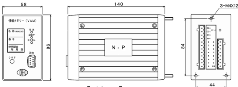
【外観図】
