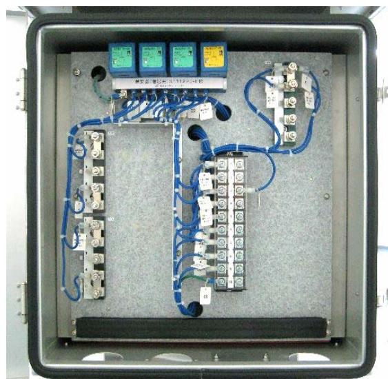
外線接続側実装写真
