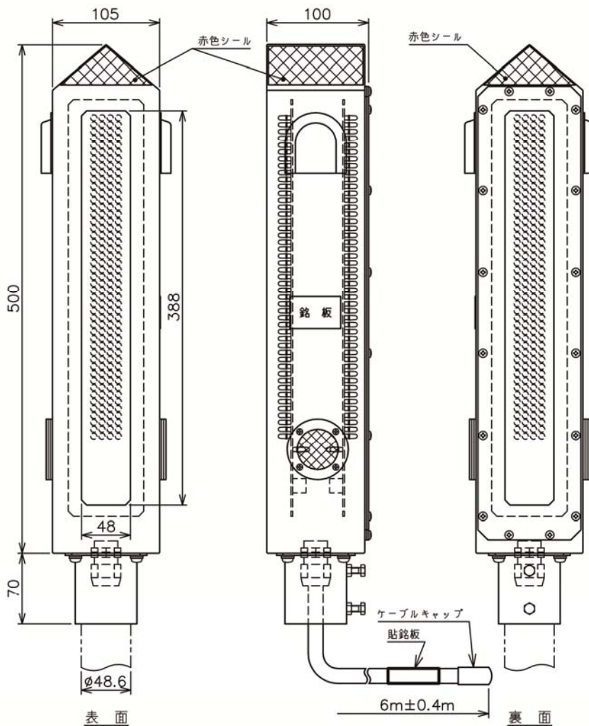
【外観図】
