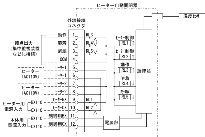
【結線図／外観図】
