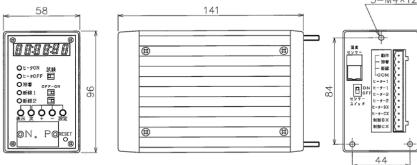
【結線図／外観図】
